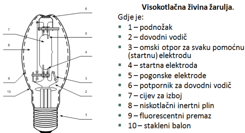
Sl. 2.6. Dijelovi visokotlačne živine žarulje, [1]
