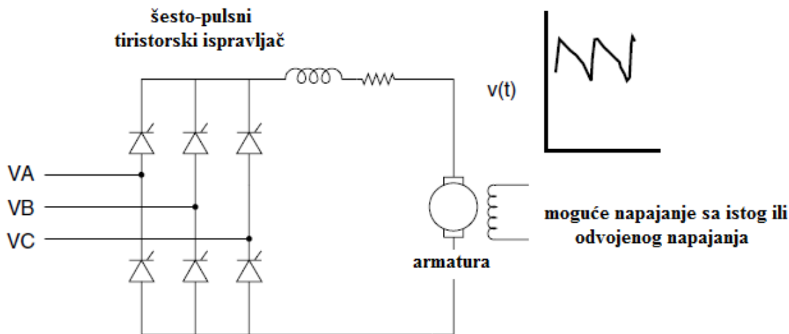
Slika 2.8. Šestero-pulsni tiristorski ispravljač [1]
