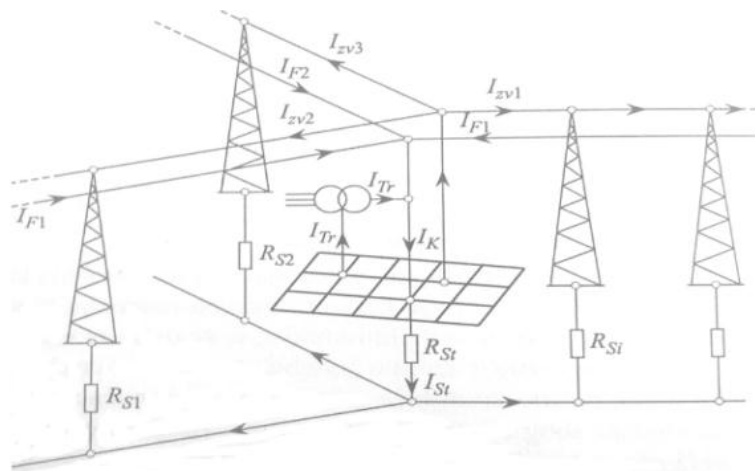
Slika 2.6) Zduženo uzemljenje [1]
