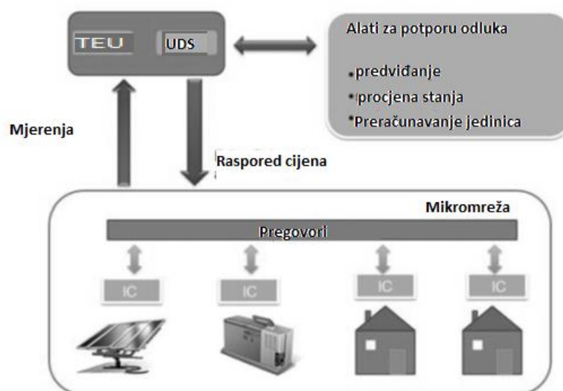
Slika 3.4. Decentralizirano upravljanje
