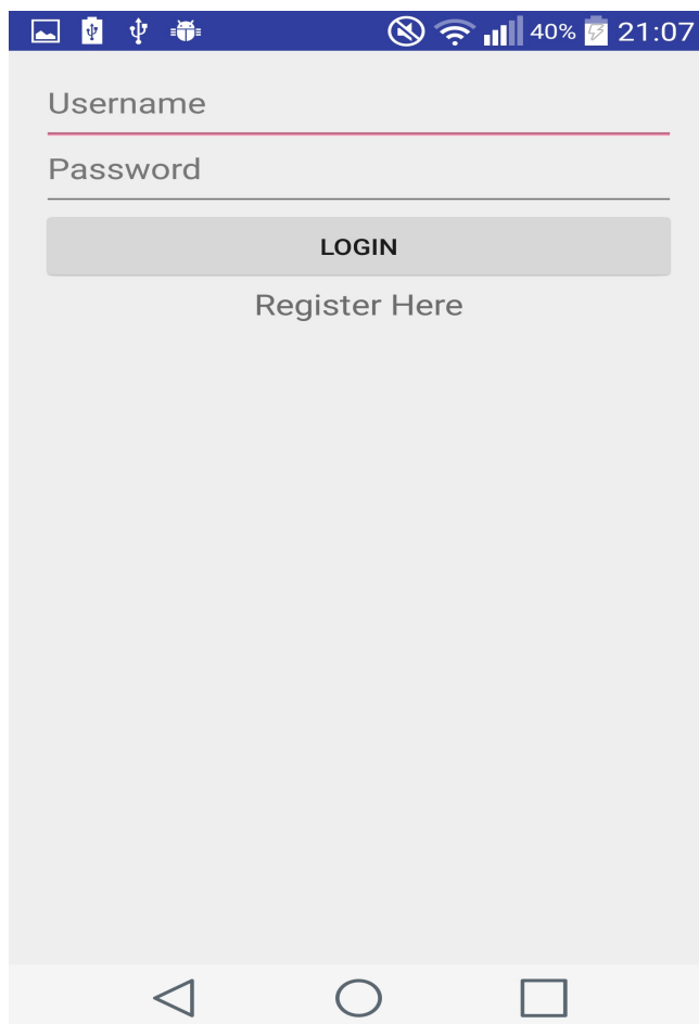
Slika 4.23. activity_login.xml
