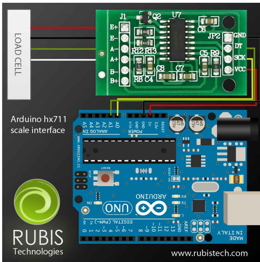
Slika 6.8. HX 711 spajanje
