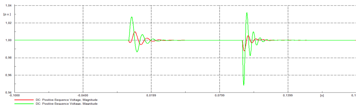
Slika 5.26 Napon na DC sabirnici STATCOM - a
