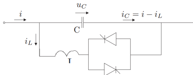
Slika 4.8. Shema TCSC –a
