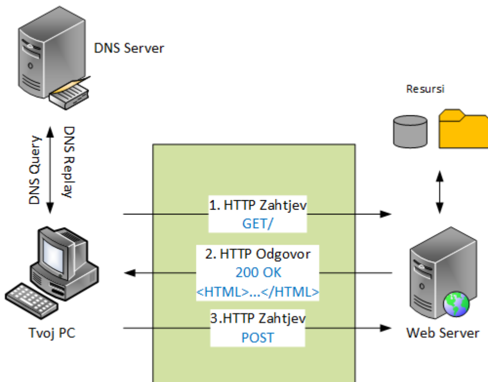
Slika 2.4.HTTP komunikacija
