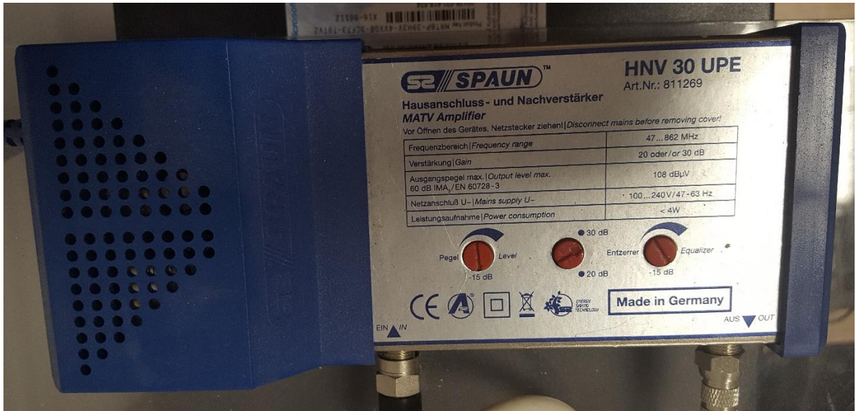
Slika 3.4 Pojačalo signala
