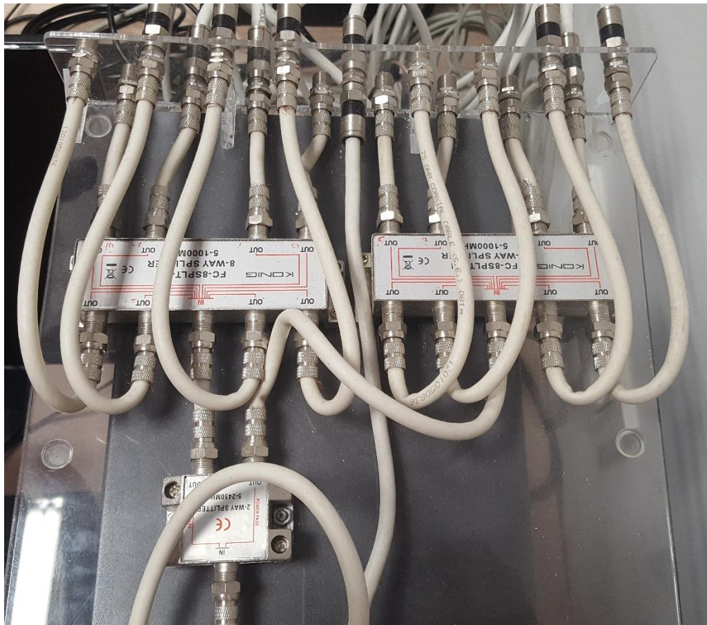
Slika 3.5 Djelitelj signala
