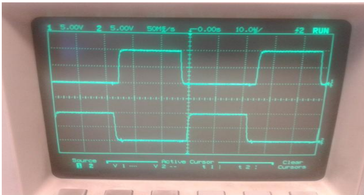
Slika 6.5 Valni oblik upravljačkog napona na upravljačkim elektrodama
