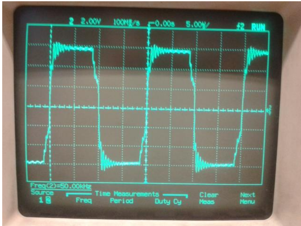
Slika 6.15 Valni oblik na trošilu
