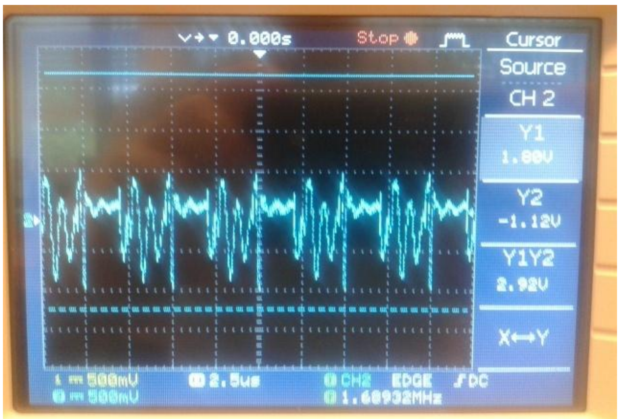
Slika 6.12 Valni oblik napona trošila
