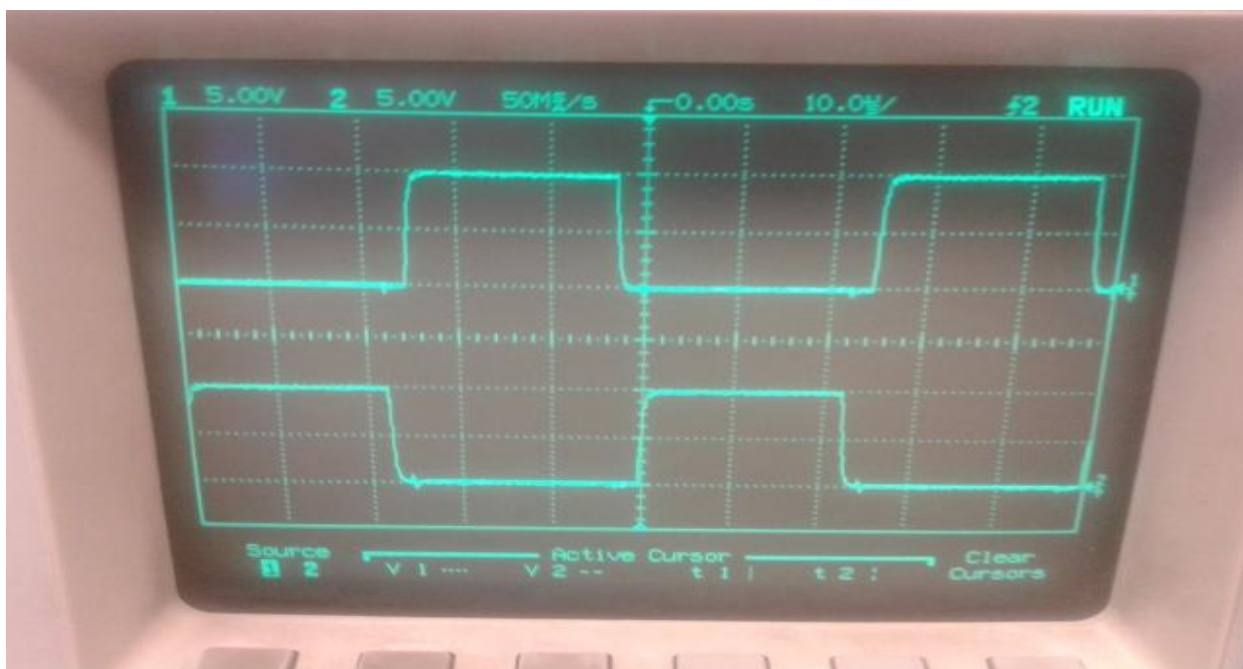
Slika 6.5 Valni oblik upravljačkog napona na upravljačkim elektrodama
