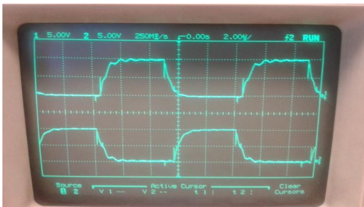
Slika 6.9 Valni oblik upravljačkog napona na upravljačkim elektrodama
