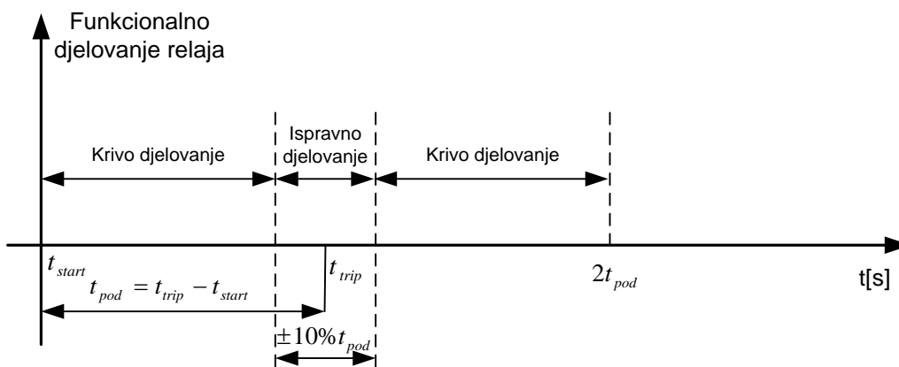
Slika 6.4: Realno ispravno djelovanje releja promatrano u vremenu
