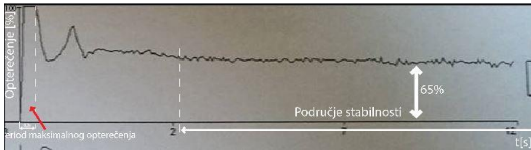
Slika 3.19. Oscilogram opterećenja alternatora bez uključenih svjetala
