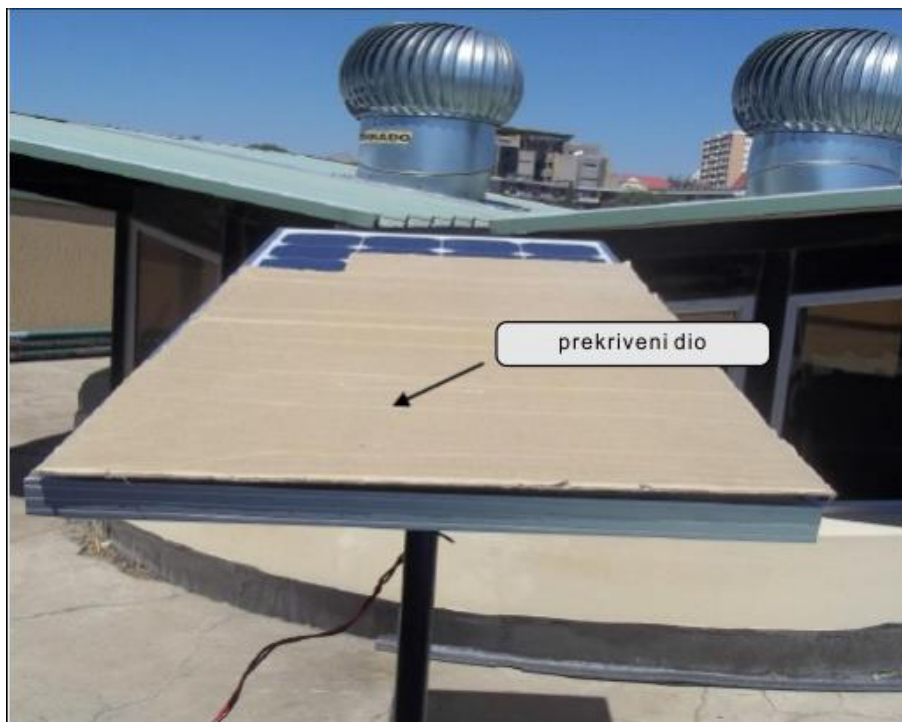
Slika 2.3. Fotonaponski modul, tri četvrtine prekrivene.
