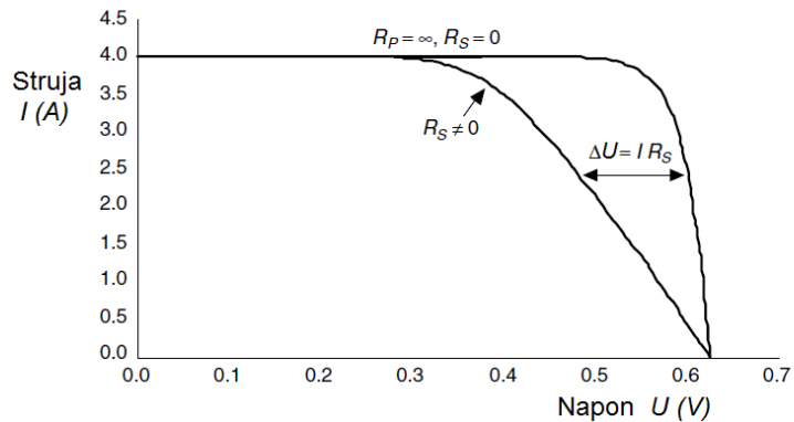
Slika 3.24. Utjecaj otpora R_S u nadomjesnoj shemi fotonaponske ćelije na izgled U-I karakteristike.
