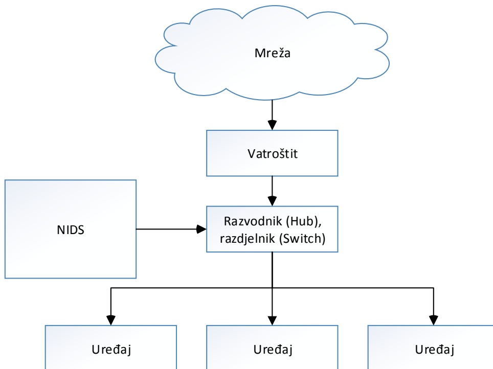
Slika 5-8. Mrežni IDS
