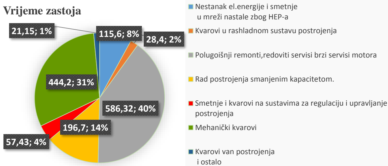
Dijagram 4.6. Omjer vremena zastoja bioplinskog postrojenja
