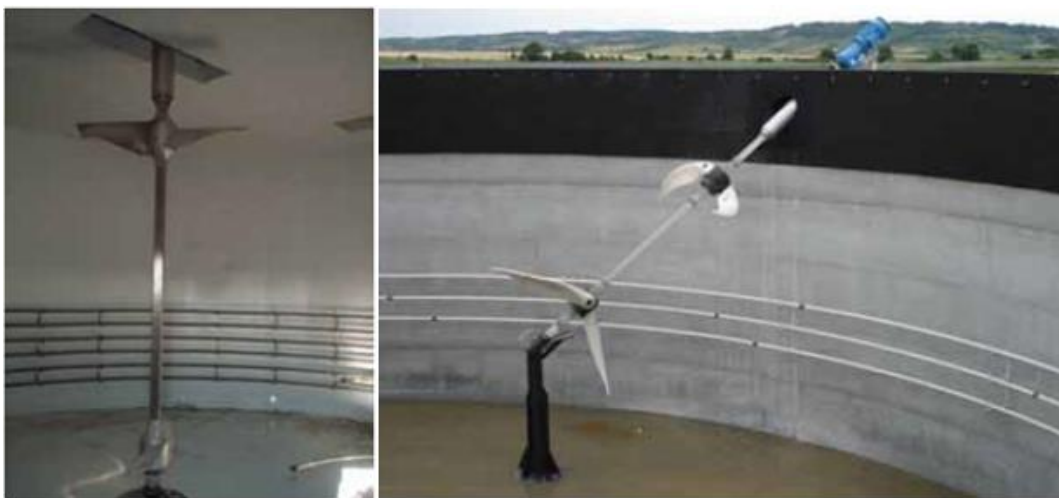
Slika 2.15. Različite vrste mješalica s lopaticama [4]
