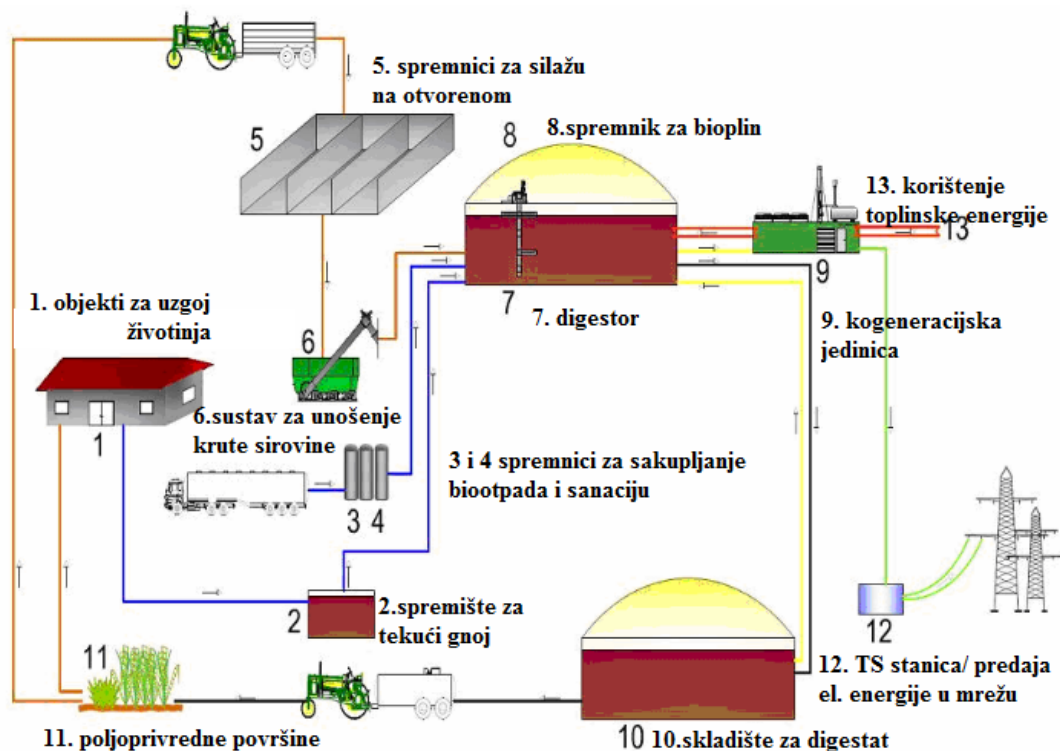
Slika 2.7. Bioplinsko postrojenje [5]
