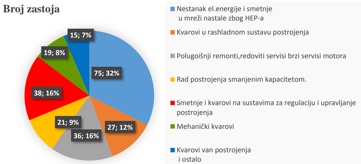
Dijagram 4.7. Omjer broja zastoja bioplinskog postrojenja
