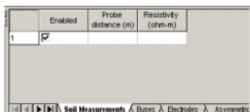
Slika 5.2. Unos podataka
