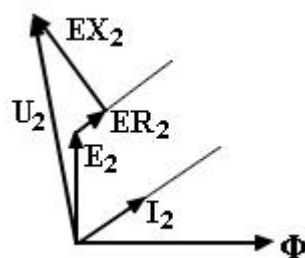
Slika 3.8. Fazorski dijagram opterećenog generatora [14]
