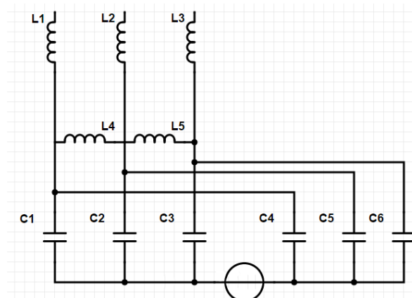
Slika 3.2. Shema zvijezda spoja pasivne kompenzacije [22]
