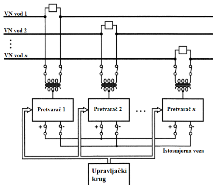
Slika 4.28. Općeniti IPFC model za n vodova [6]
