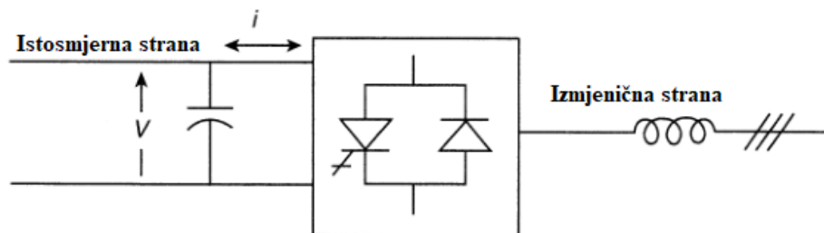
Slika 4.27. Model STATCOM-a [6]
