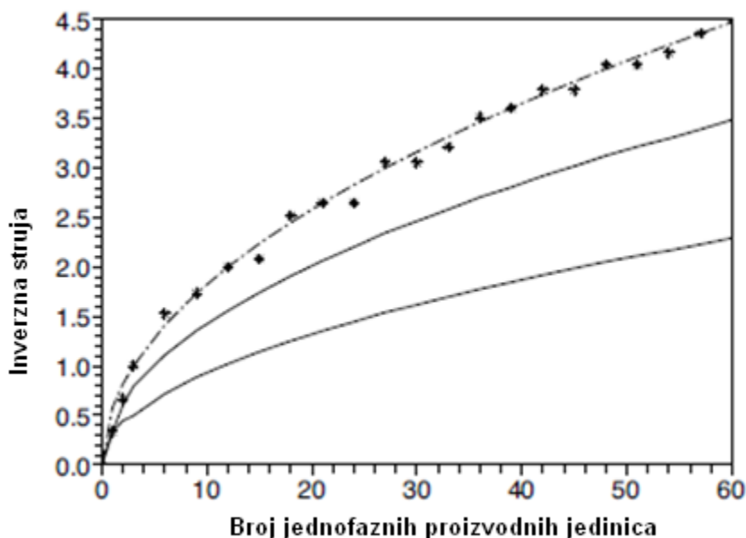
Slika 5.3 Inverzna struja uzrokovana povećanjem broja jednofaznih proizvodnih jedinica[4]
