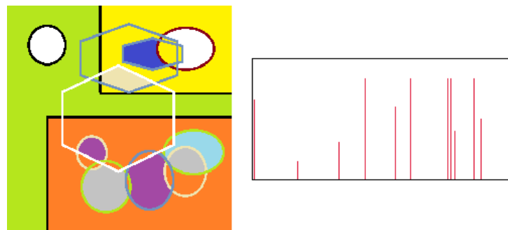
Slika 2.4. Histogram slike
