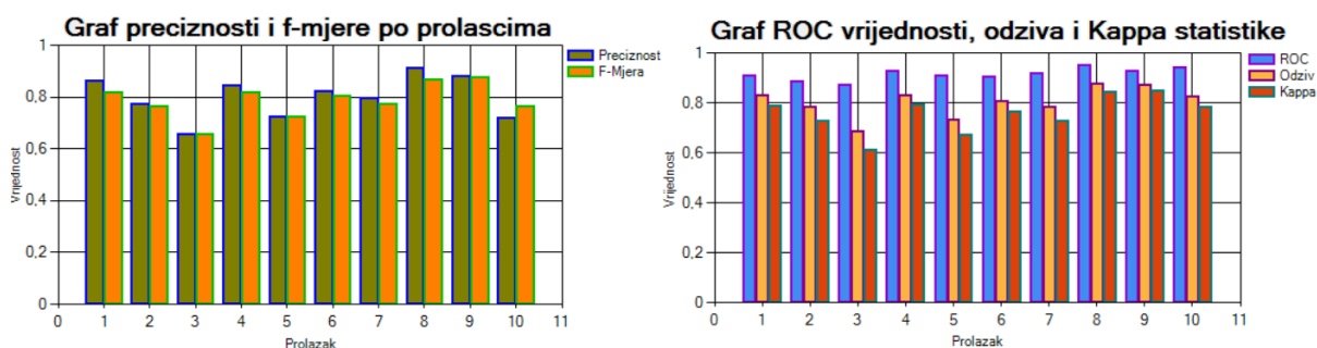
Slika 3.14. Rezultati po prolascima za SVM klasifikator, Cohn-Kanade baza
