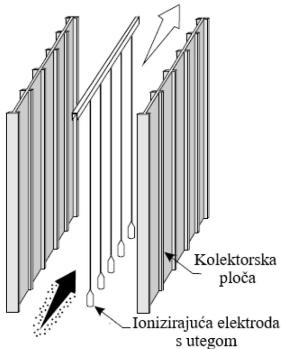
Sl. 3.1. Pločasto-žičani ESP
