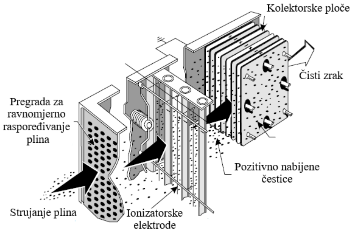
SI 3.3. Dvostupanjski ESP
