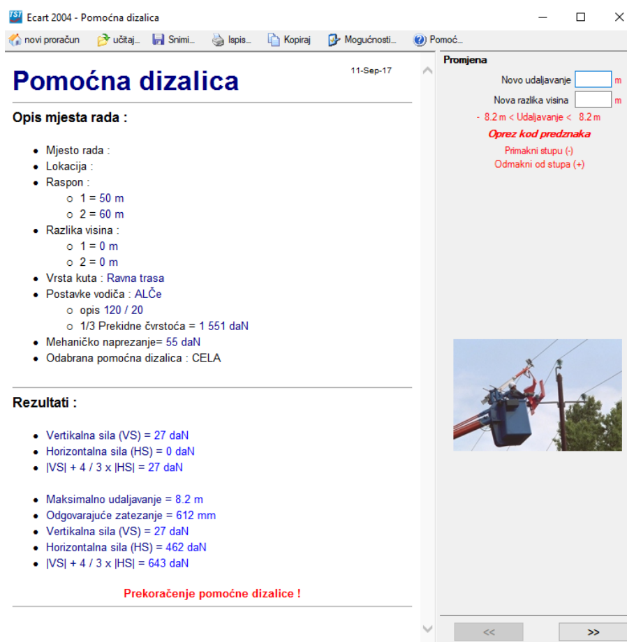
Sl. 4.3. Proračun dodatnog napreznjanja vodiča pomoću „ECART 2004“ programske podrške
