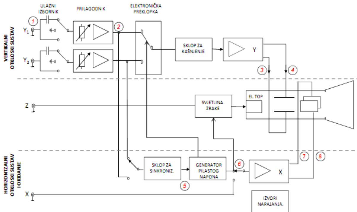
Sl.3.2. Blok shema dvokanalnog analognog osciloskopa [11]
