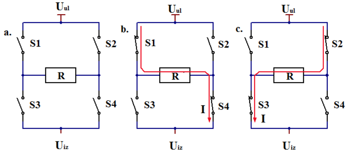
Slika 4.3. Prikaz H-mosta [11]
