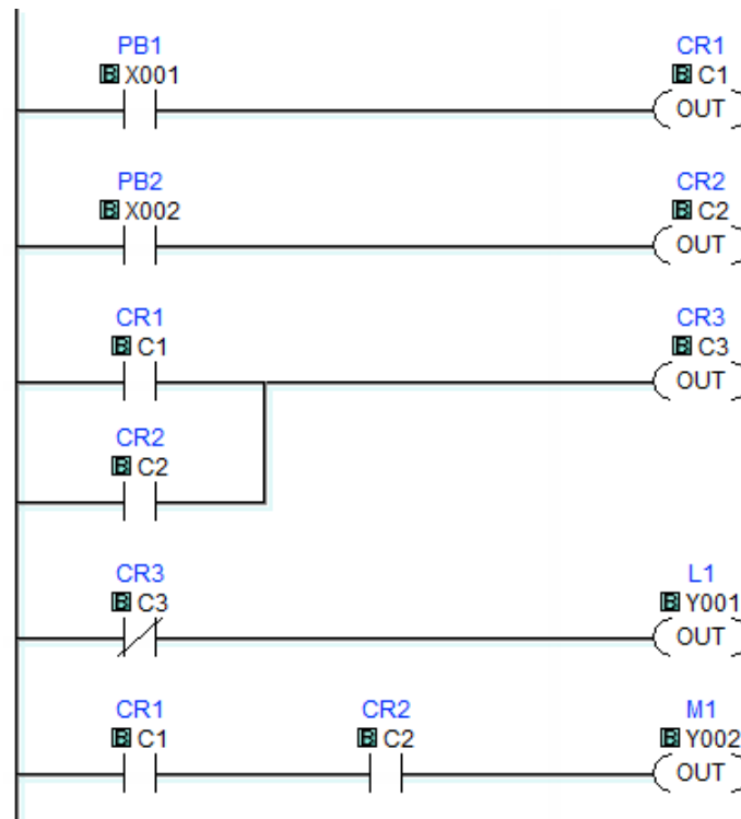
Slika 5.3. Ljestvena logika PLC-a [16]
