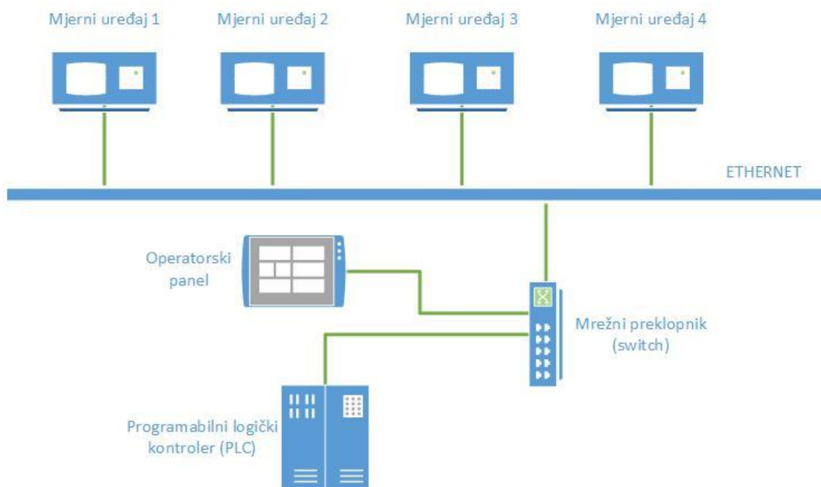
Slika 3.15. Blok shema
