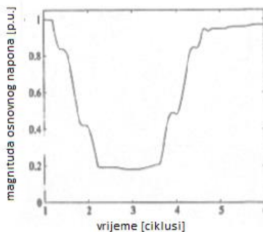
Slika 4.6. Magnituda komponente osnovnog napona naponskog propada [9]
