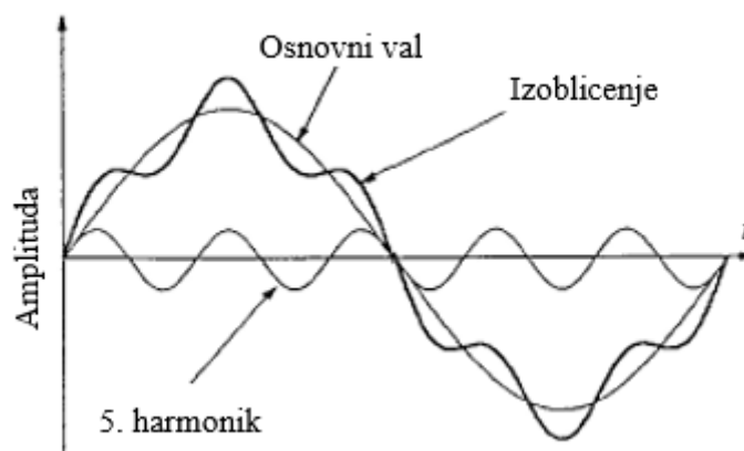
Slika 3.6. Izobličeni sinusni val [10]
