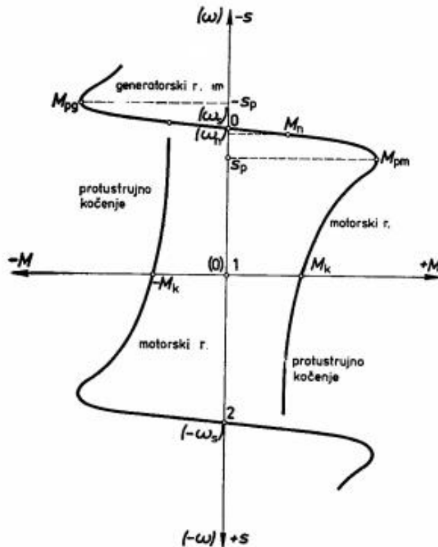
Slika 2.4. Mehanička karakteristika pri različitim smjerovima vrtnje [3]
