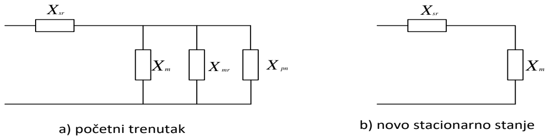
Sl. 2.6. Reaktancije generatora za vrijeme kratkog spoja
