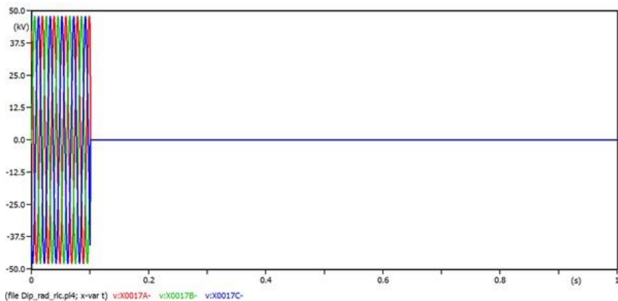
Sl. 5.14. Valni oblici napona pojedinih faza na mjestu kvara pri trofaznom kratkom spoju
