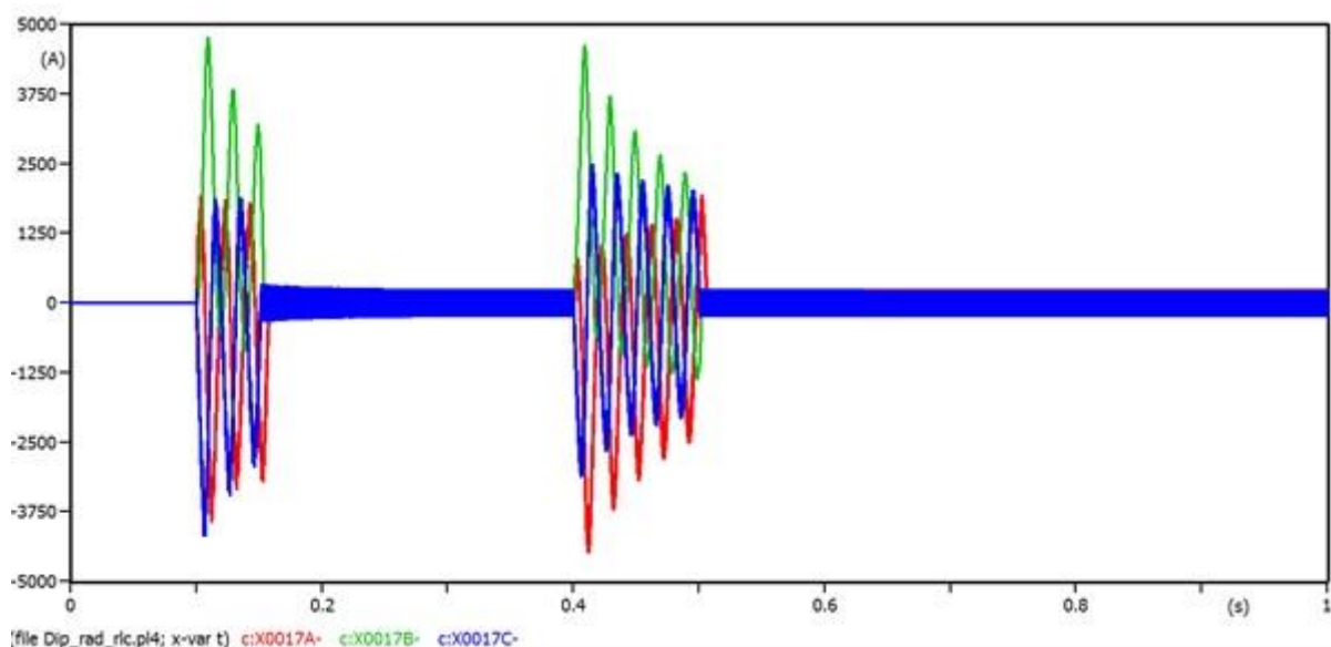
Sl. 5.15. Valni oblici struja pojedinih faza na mjestu kvara pri trofaznom kratkom spoju
