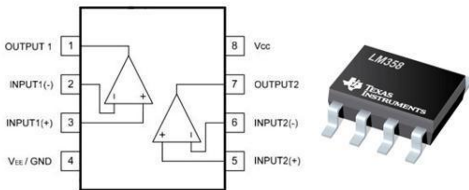
Sl. 2.5. LM358
