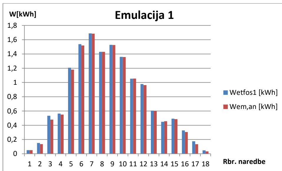
Slika 4.6. Odnos stvarnog i emuliranog dijagrama proizvodnje
