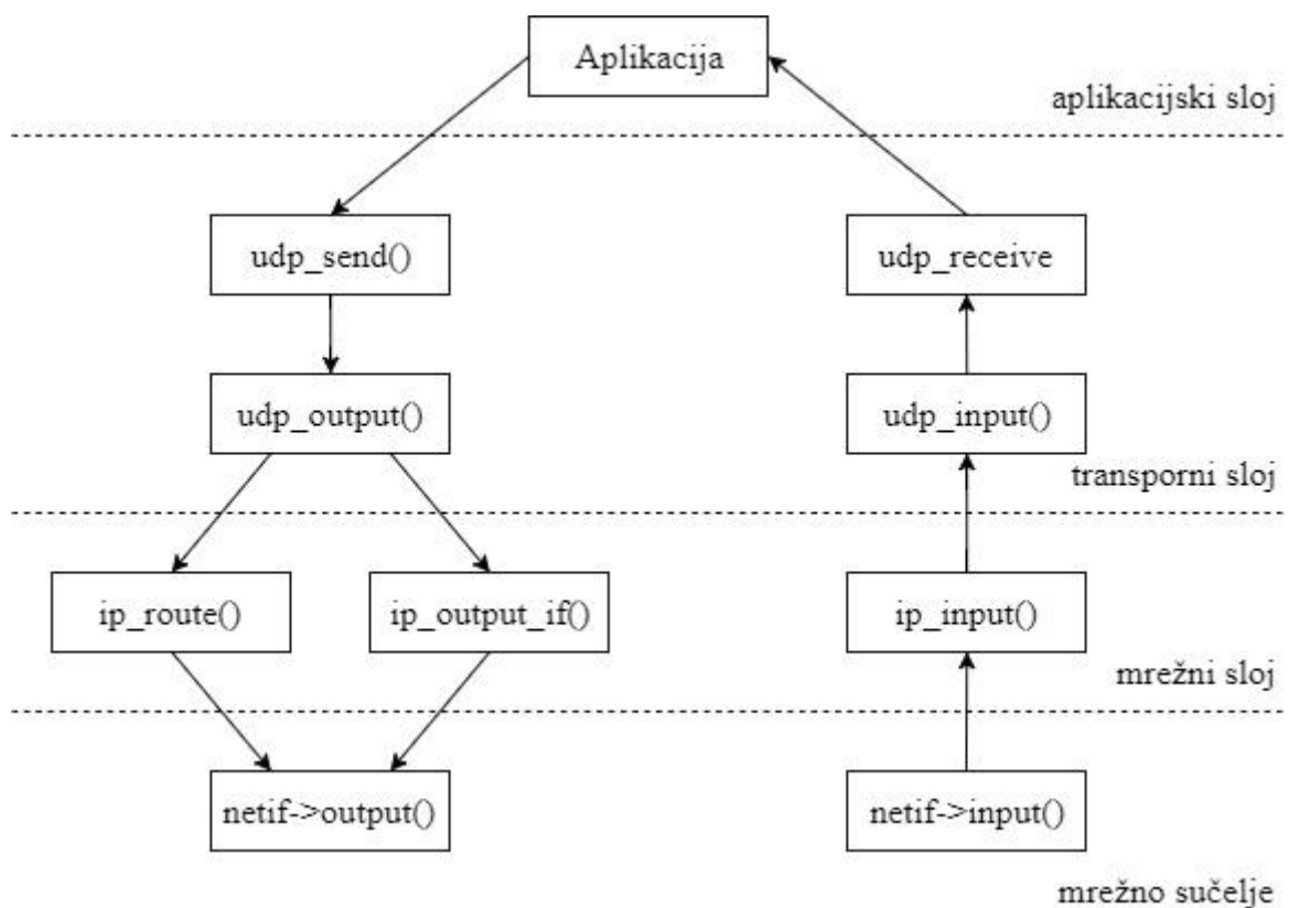
Slika 3.15. Arhitektura lwIP-a [3]
