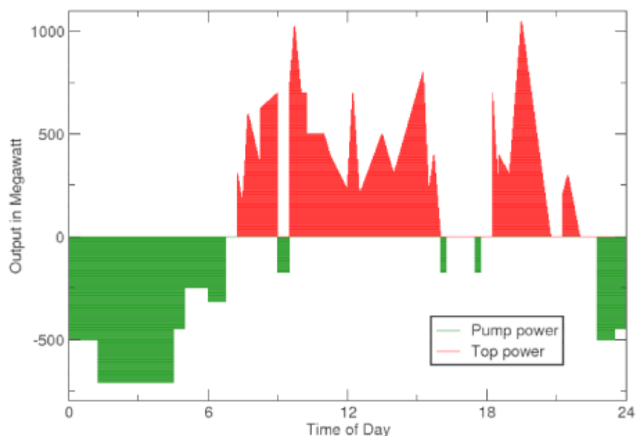
Sl. 4.5. Tipični dnevni režim rada crpno-akumulacijske elektrane [15]
