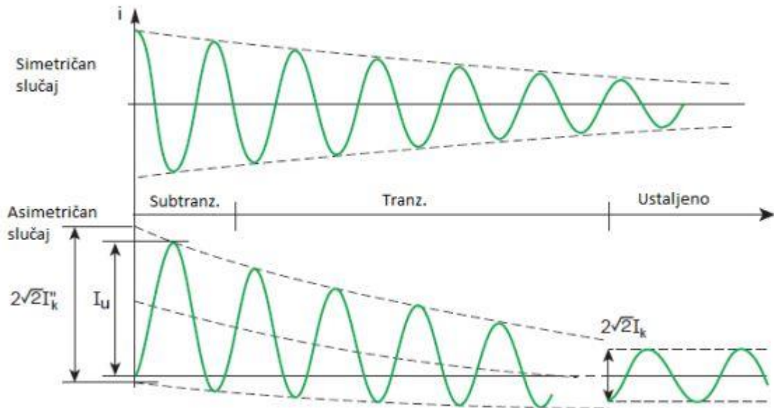
SI.3.5. Kratki spoj blizu generatora za simetričan i asimetričan slučaj [8]
