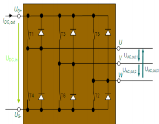
Slika 3.8. Izmjenjivač s ekvivalentnim sklopama
