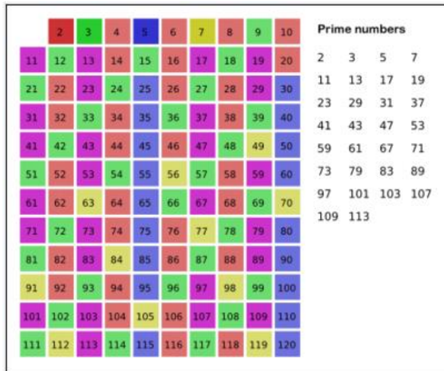
Sl. 3.5. Oznacavanje svih prostih brojeva [9].
