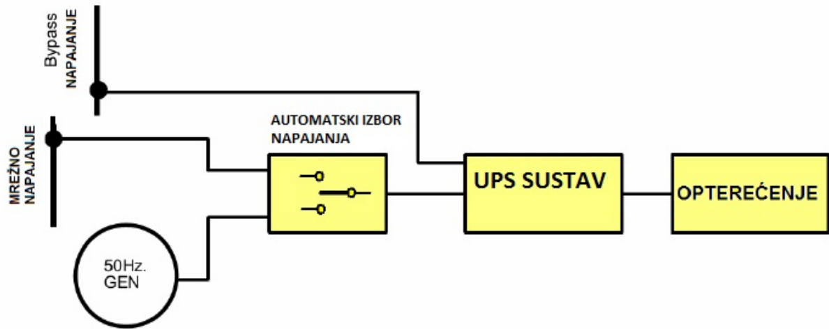
Slika 4.10. Aktivni UPS sustav sa agregatom, odvojeni bypass [2]
