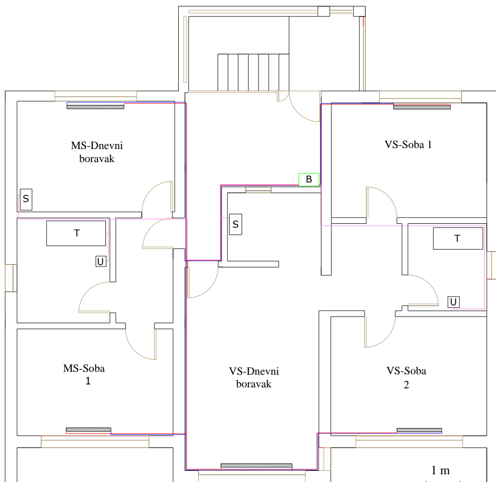
Slika 4.10. Tlocrt kata sa instalacijom centralnog grijanja i PTV-a.
