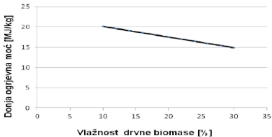
Slika 3.8. Ovisnost donje ogrjevne moći drvne biomase o vlažnosti [7]
