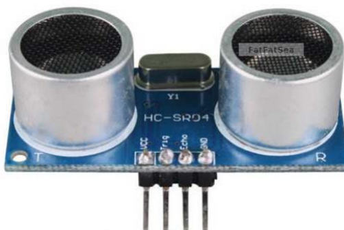
SI 3.9. HC-SR04 [10]
