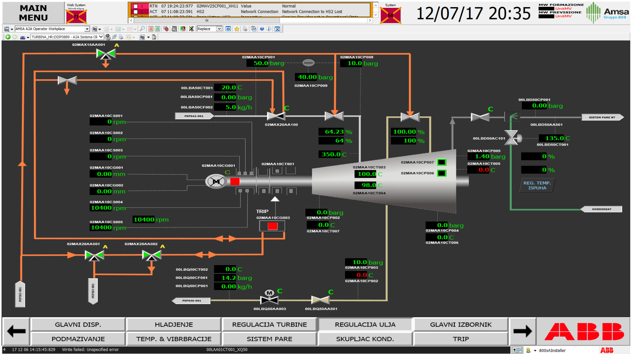
Slika 7.7 Regulacije ulja
