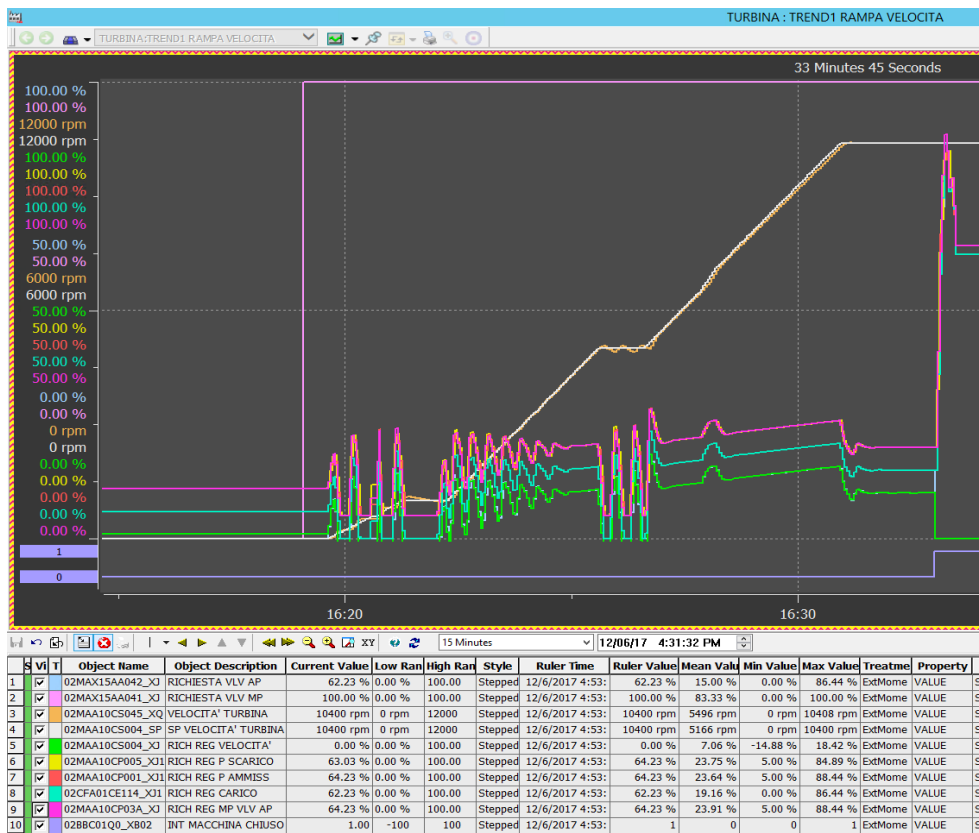
Slika 7.2 Trend regulacije
