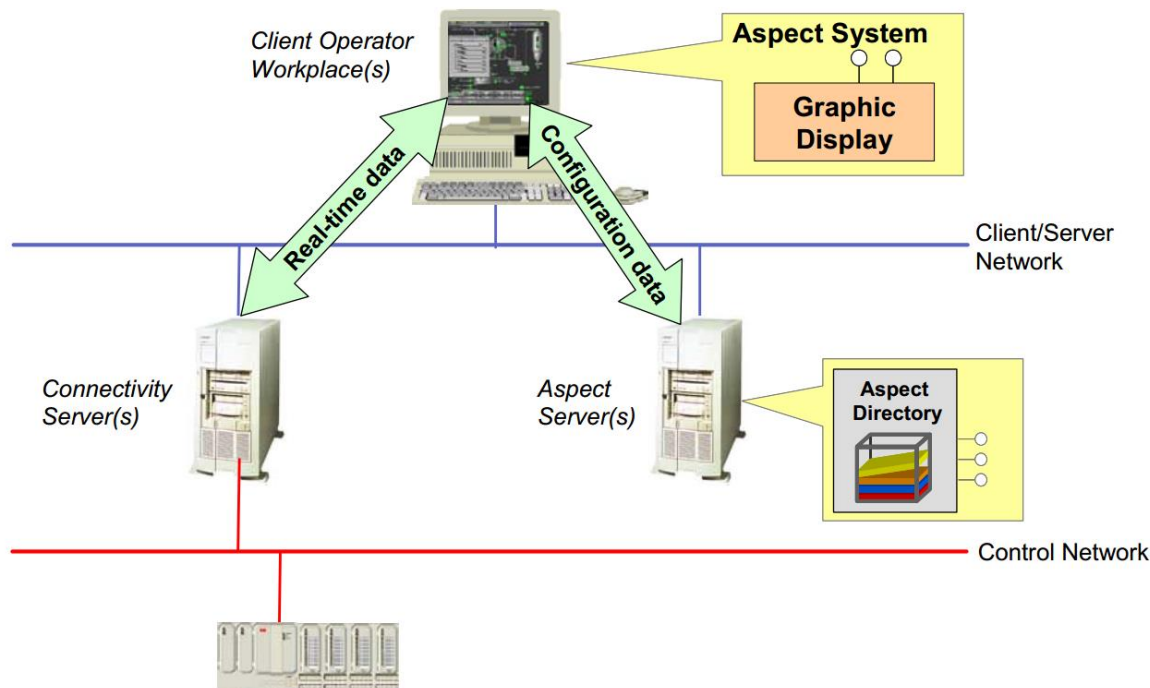
Slika 3.18 Vizualizacija objekata
