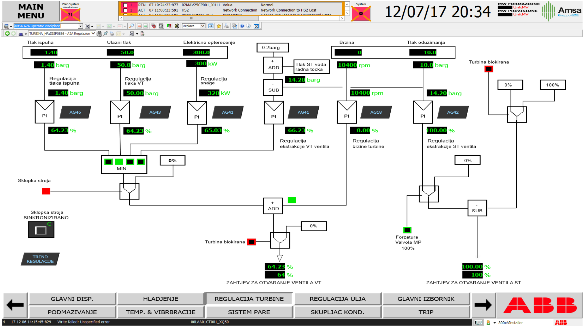
Slika 7.5 Regulacija HMI
