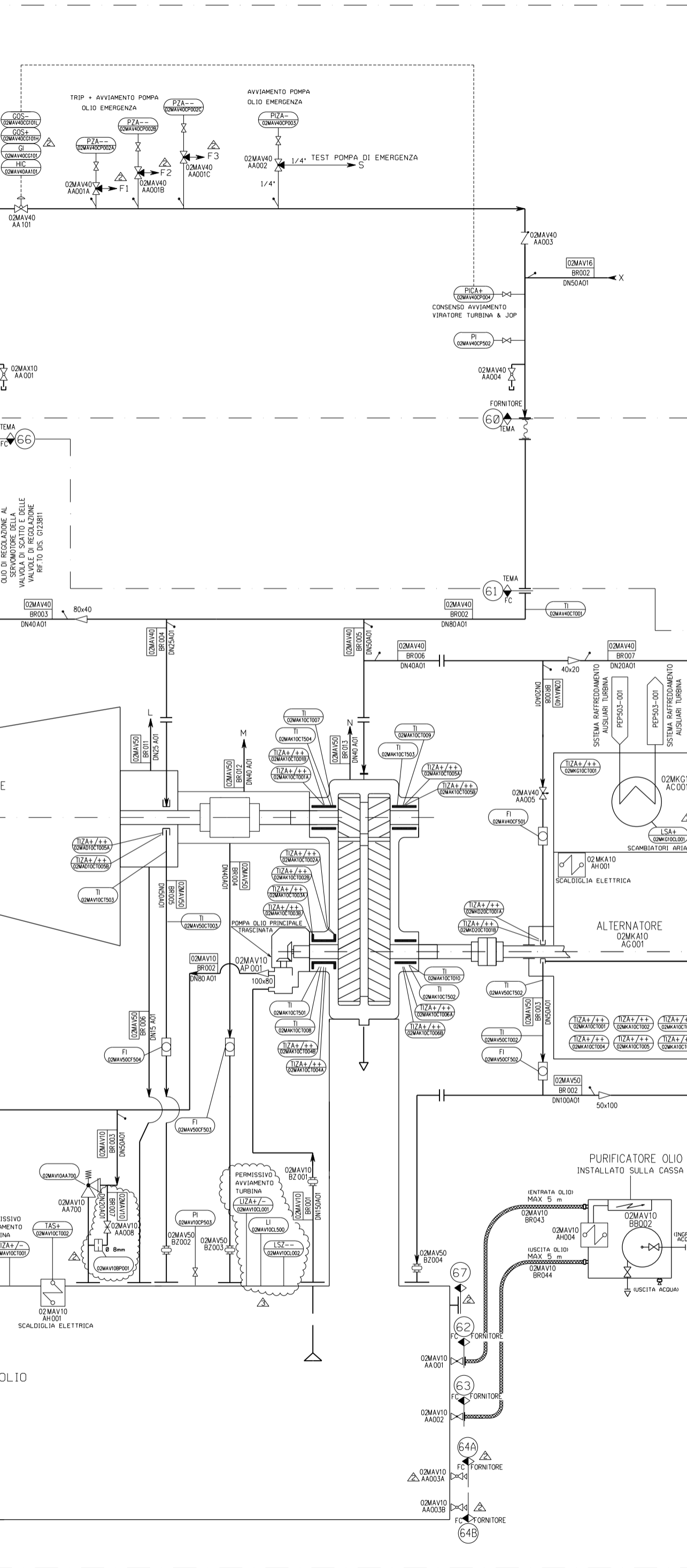
Slika 4.2 P&ID Sustav podmazivanja 2/2
