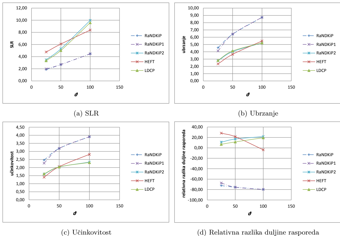
Slika 5.21: Testni slučajevi iz repozitorija Pegasus za različit n , raznorodna komunikacija.
