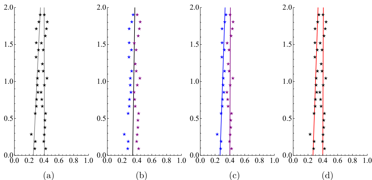
Slika 4.3: Primjer rada algoritma 2. (a) Referentni redovi usjeva i generirane točke, (b) TLS pravac, (c) Pravci dobiveni primjenom DIRECT algoritma, (d) Pravci dobiveni nakon korekcije k -means algoritmom (algoritam 1).
