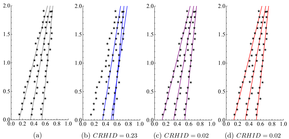
Slika 7.7: Primjer pokusa prepoznavanja tri reda usjeva u slučaju potpunog zasijanja i veće varijance ( \sigma^2 = 0.02 ). (a) Generirane točke, (b) HT metoda, (c) IMLD metoda, (d) CRDI metoda.
