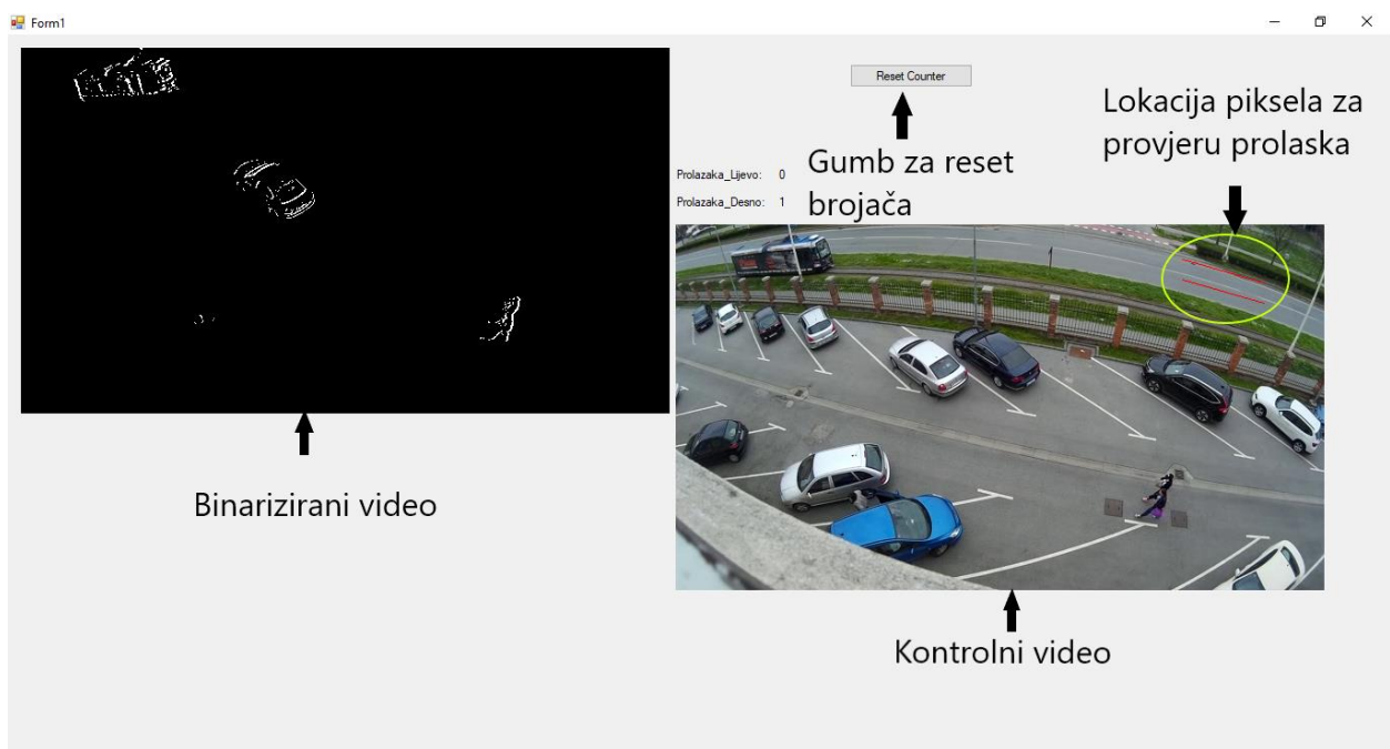
Slika 4.1. Grafičko sučelje
