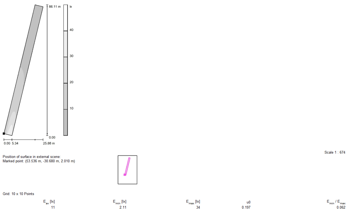
Slika 4.6 Numerički rezultat generiran svjetlotehničkim proračunom u DIALuxu koristeći proračunsko polje kako bi se iskazale vrijednosti razina osvijetljenosti duž slapa
