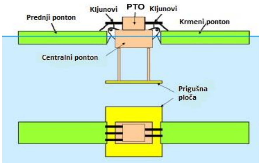
SI. 3.28. Prikaz McCabe-ove valne pumpe
