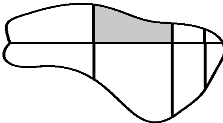
Sl 2.4 Cijepanje nepravilnog ravninskog lika na krivoljne trapeze
