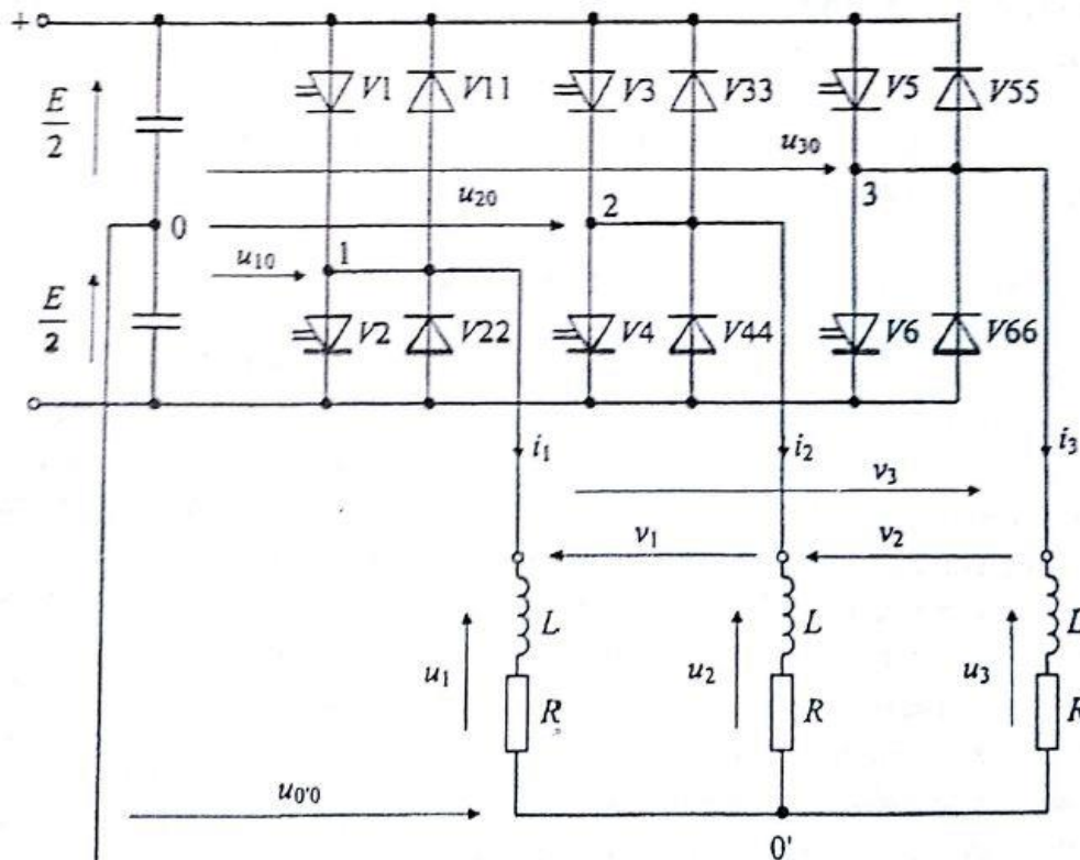
Slika 3.1 Shema spoja izmjenjivača u trofaznom mosnom spoju s označenim referentnim smjerovima napona i struja trošila prema srednjoj točki
