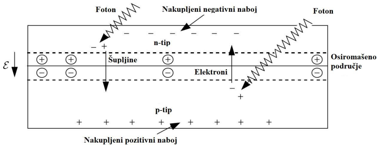
Slika 3.3 Fotonaponska ćelija [9]
