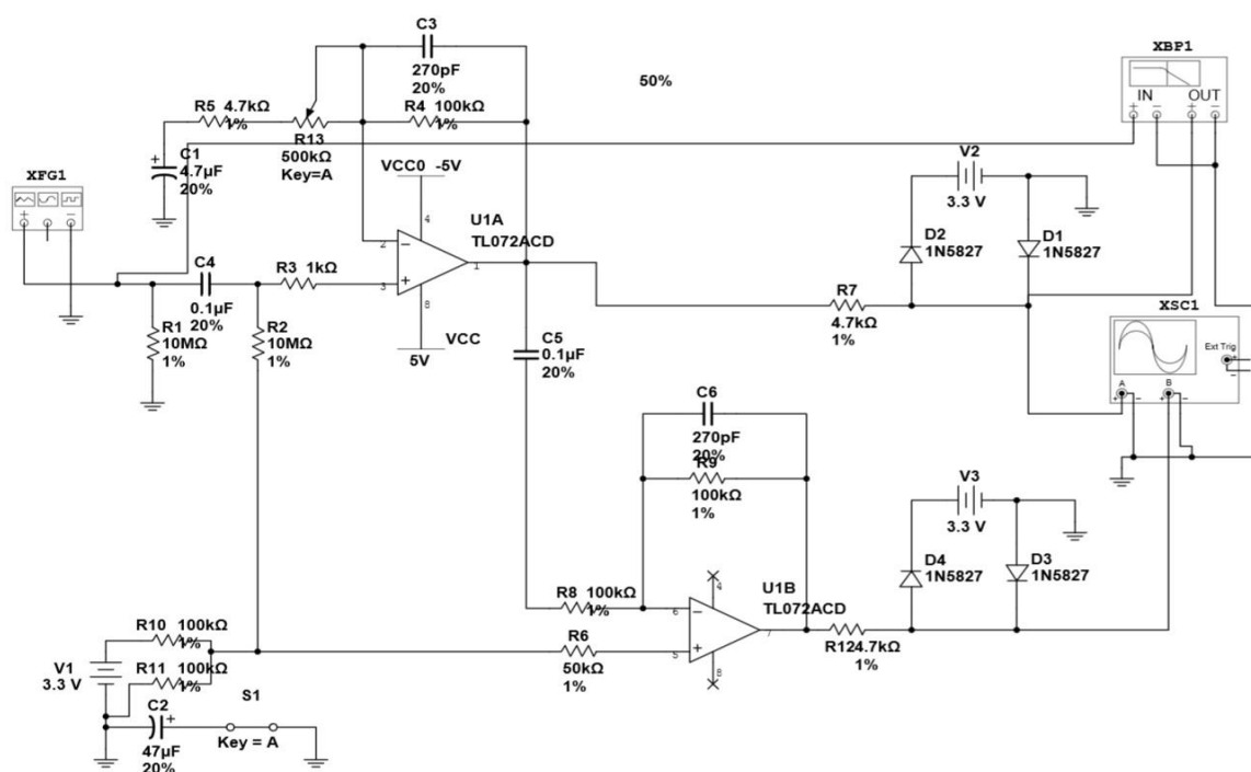
Slika 3.4. Model pred-pojačala
