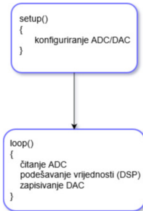
Slika 4.1. Arhitektura programa
